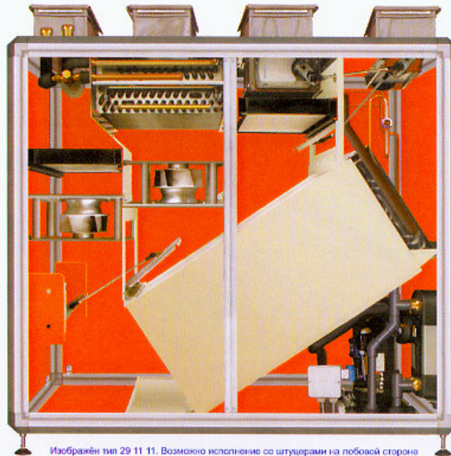
Изображен тип 29 11 11. Возможно исполнение со штуцерами на лобовой стороне
